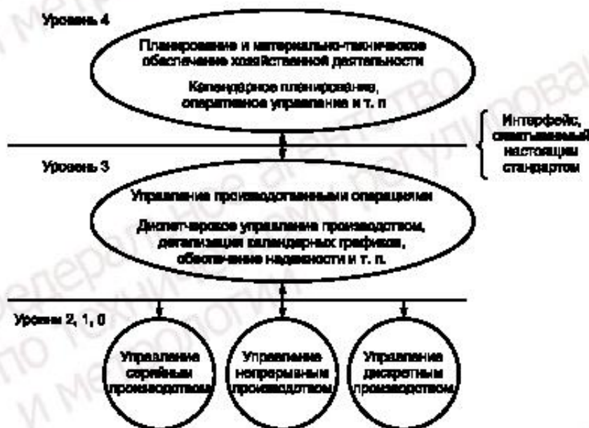
Рисунок 3 — Функциональная иерархия
