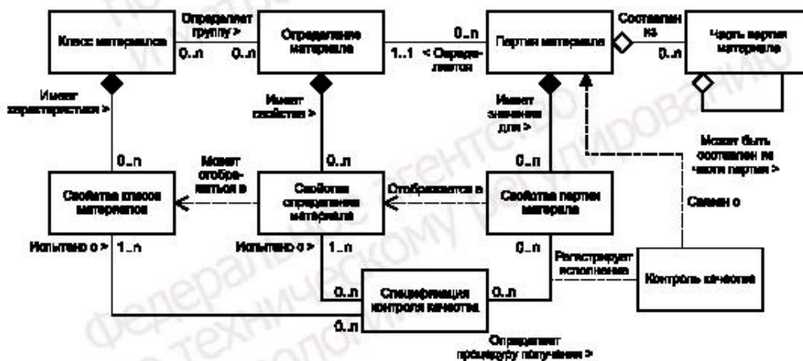
Рисунок 16 — Модель материалов
