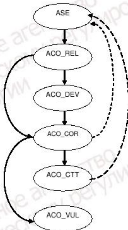
Рисунок 17 – Взаимосвязь между семействами класса АСО
