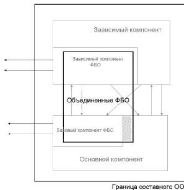
Рисунок В.3 – Обобщенное представление составного ОО
