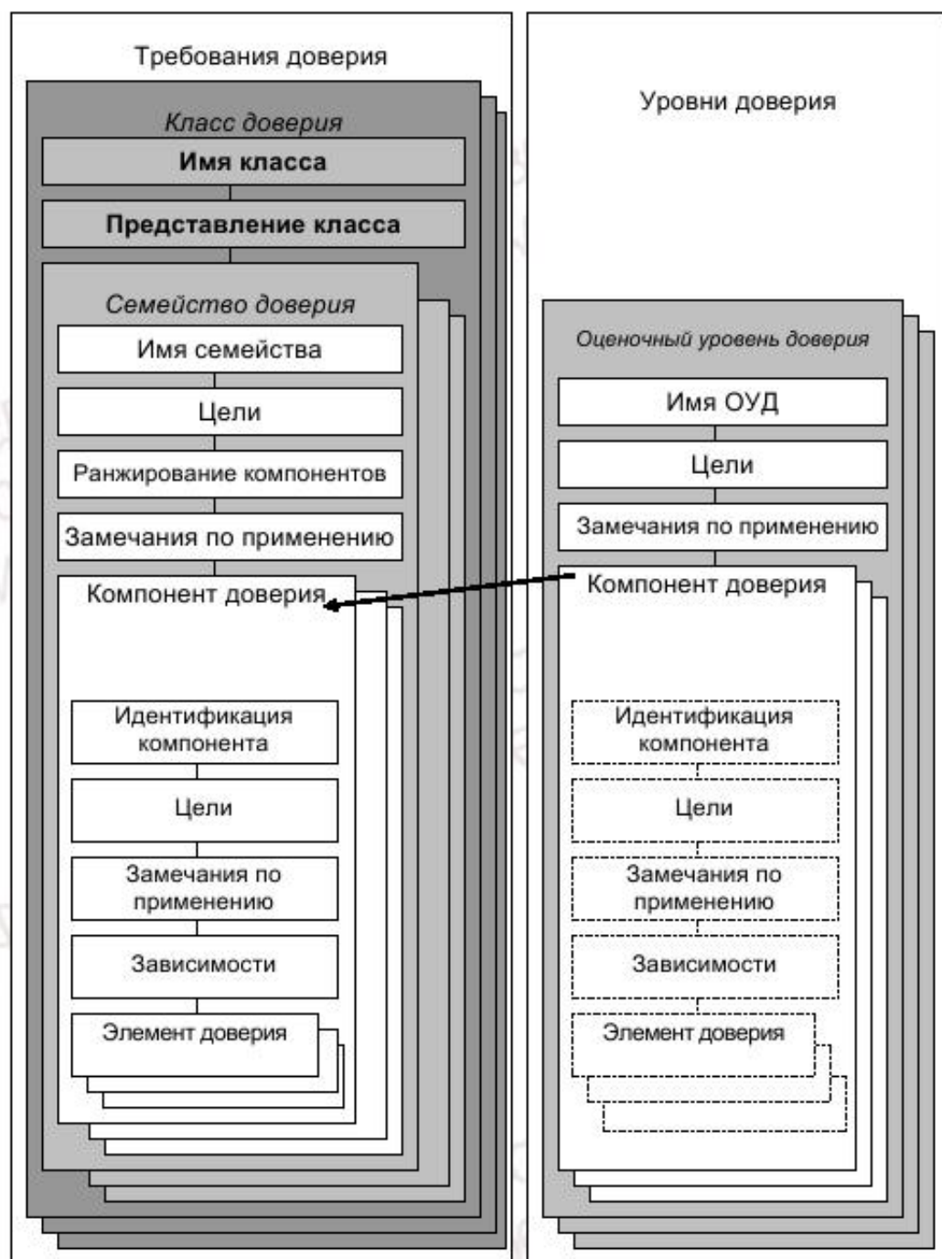
Рисунок 5 – Взаимосвязь требований и уровня доверия
