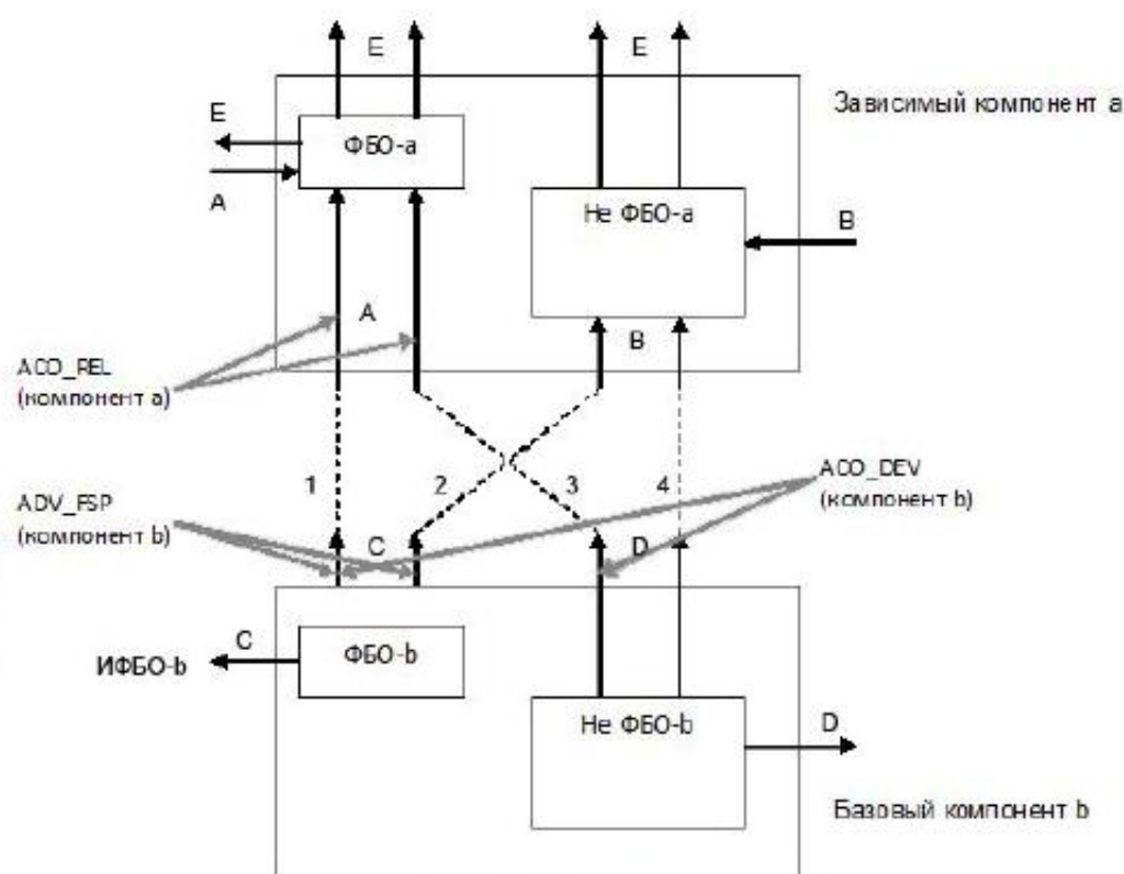
Рисунок В.4 – Взаимодействие объединенных компонентов
