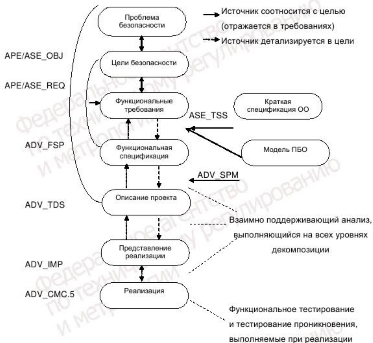
Рисунок 10 – Взаимосвязи между компонентами класса ADV и с другими семействами
