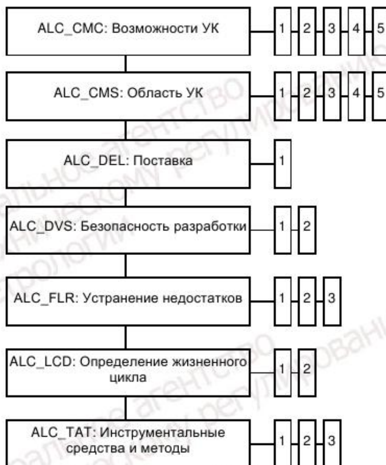
Рисунок 13 – Декомпозиция класса ALC «Поддержка жизненного цикла»
