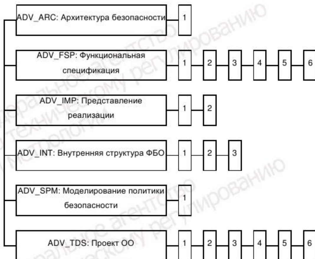
Рисунок 11 – Декомпозиция класса ADV «Разработка»
