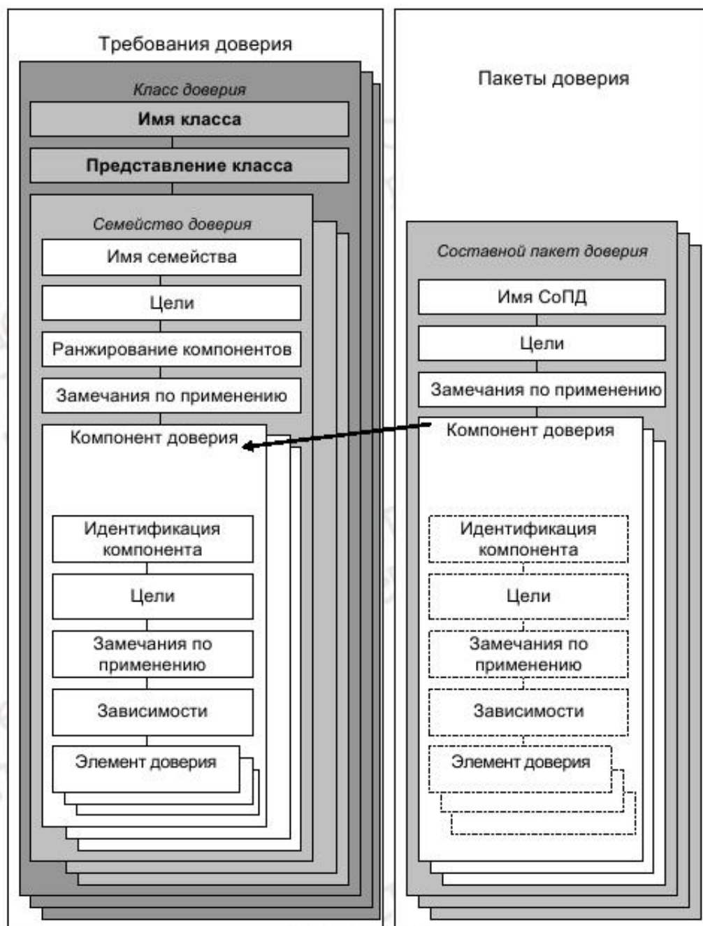
Рисунок 7 – Взаимосвязь между требованиями доверия и составными пакетами доверия
